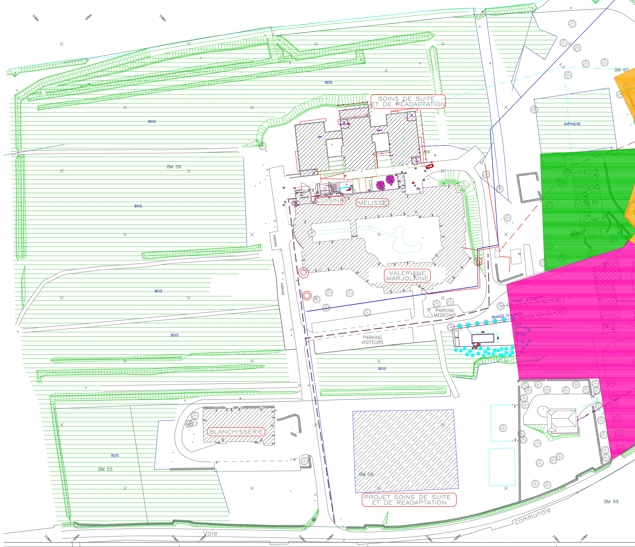
CENTRE HOSPITALIER DE LOCHES SITE DE PUYGIBAULT PLAN MASSE
