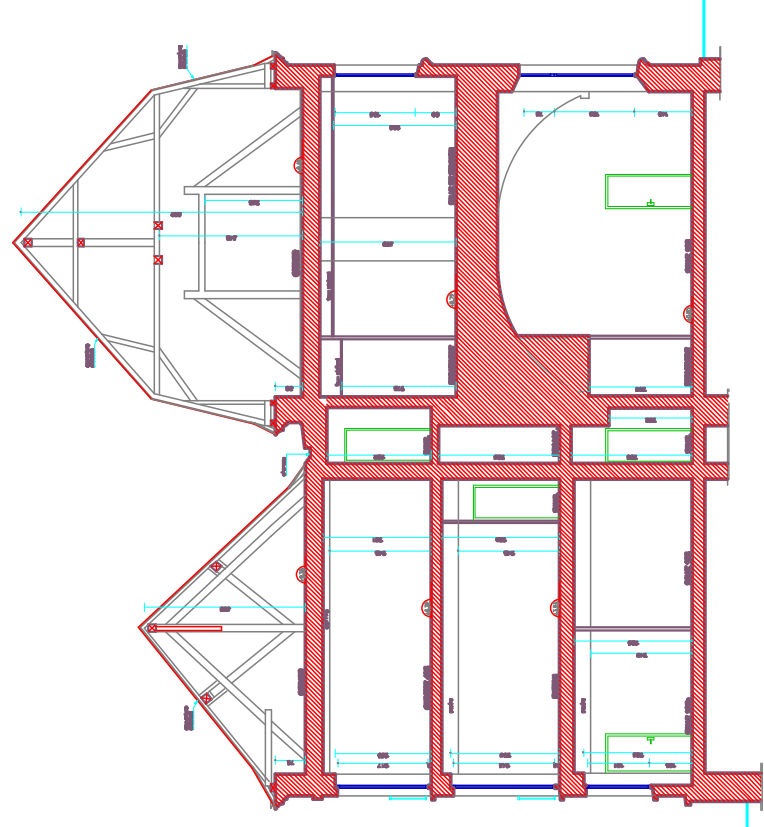
COUPE A - A
